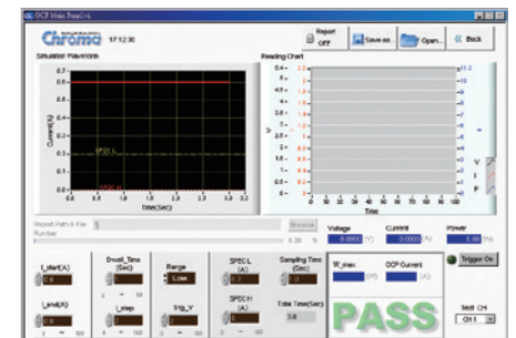
过电流保护测试
